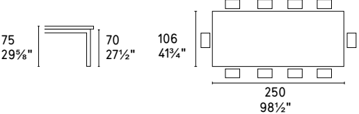
CS/4104-RL B 250
