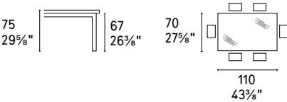
CS/4089-FMV 110
