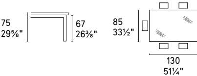
CS/4089-FMV 130
