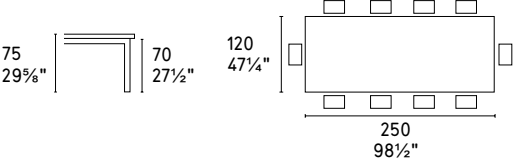
CS/4072-FRL B 250
