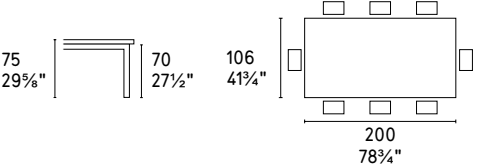
CS/4072-FRL B 200
