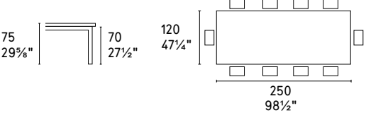
CS/4104-RL B 250
