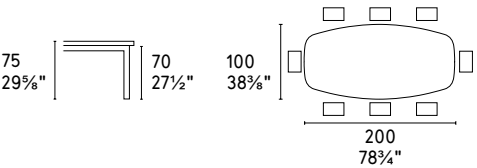
CS/4072-FEL 200
