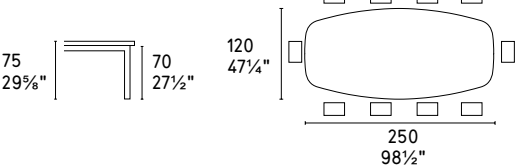
CS/4072-FEL 250
