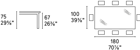
CS/4089-FMV 180
