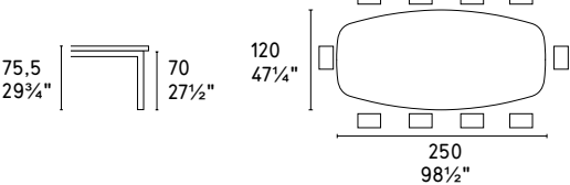
CS/4072-FRC 250
